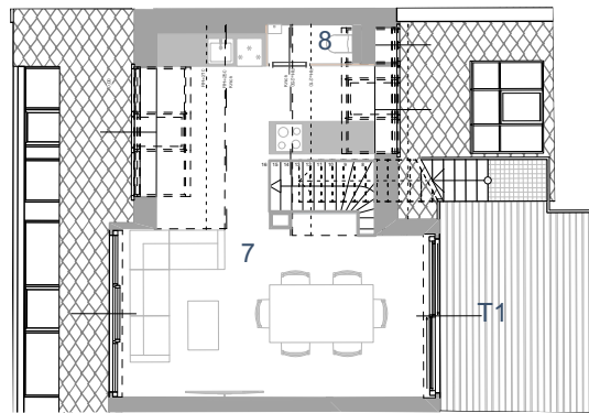
2. Dachgeschoss
