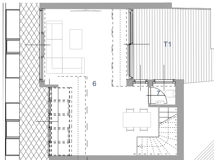
2. Dachgeschoss
