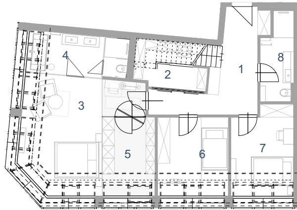
1. Dachgeschoss
