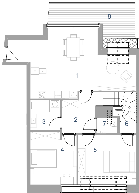
1. Dachgeschoss
